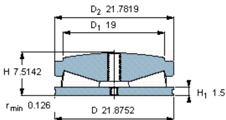
球面垫圈的半径 R 1270
