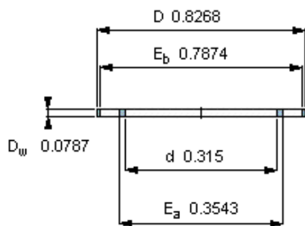
AXK 0821 TN
