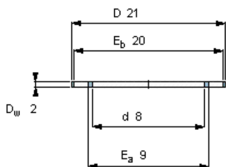
AXK 0821 TN
