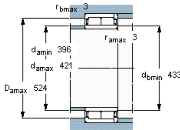
计算系数 k_r 0,2
